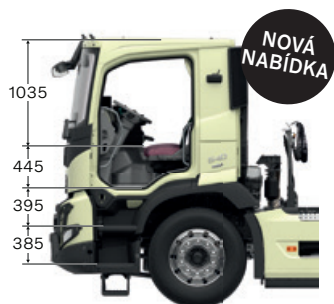
NÍZKÁ DENNÍ KABINA
