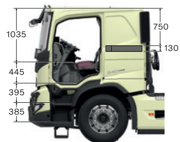
NÍZKÁ SPACÍ KABINA
